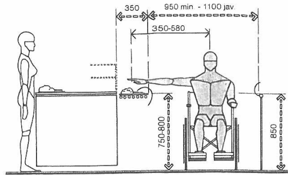
Önkiszolgáló pult méretei
