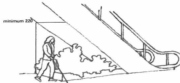
mozgólépcső, lépcsőkar 220 cm-es belmagasság alatti terének elkerítése
