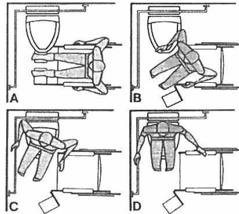
Sarok WC használata Fix kapaszkodókkal
