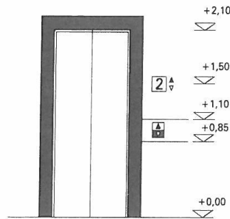
Felvonó gombok, feliratozások
