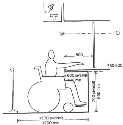
Információs pult kialakítása
