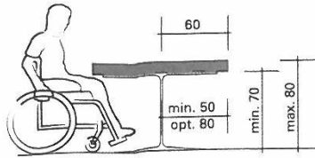
Étkezőasztal méretei
