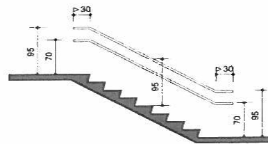
lépcső
