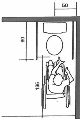
WC kialakítások, helyigények Fix/lehajtható kapaszkodókkal
