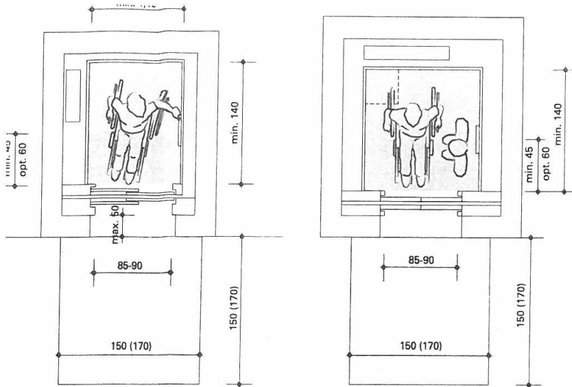
felvonó kabin helyszükségelei, helyigények az ajtó előtt
