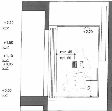
felvonó kabin
