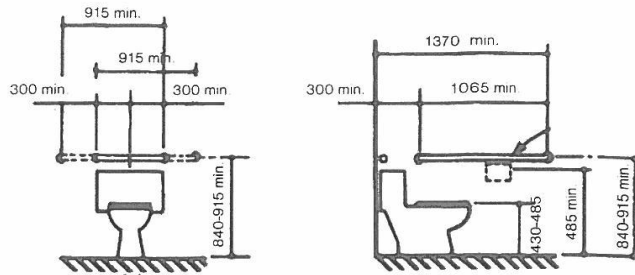
WC szerelési magasságok fix kapaszkodókkal
