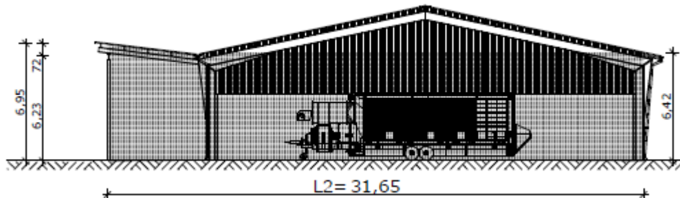
A nyugati, meglévő tároló épület metszete
