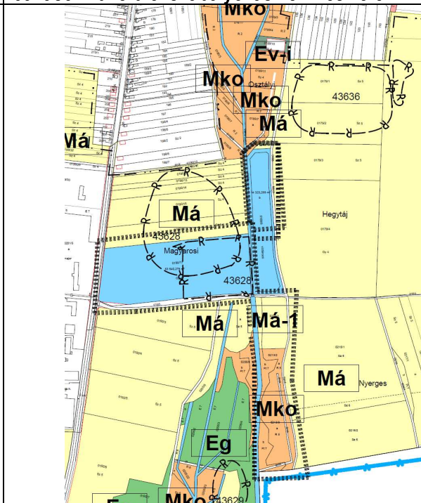
Javasolt külterület szabályozási terv részlete
