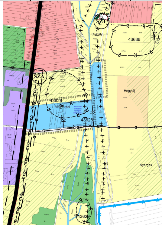
Javasolt külterület szabályozási terv részlete
