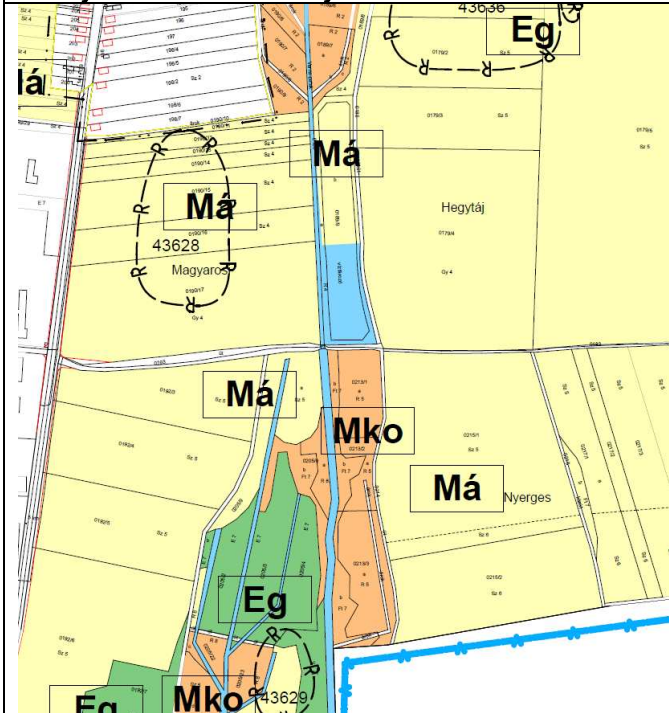
Hatályos külterület szabályozási terv részlete
