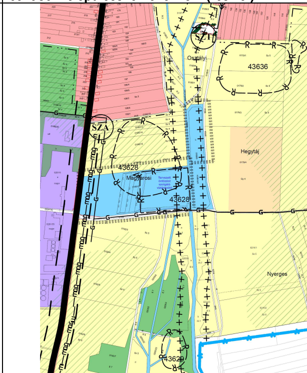
Javasolt külterület szabályozási terv részlete
