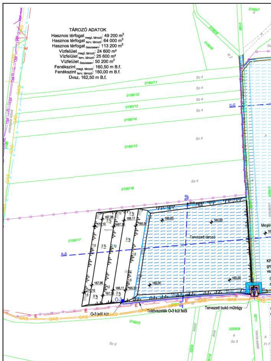
A 0190/17 hrsz öntözőtő helyszínrajza
