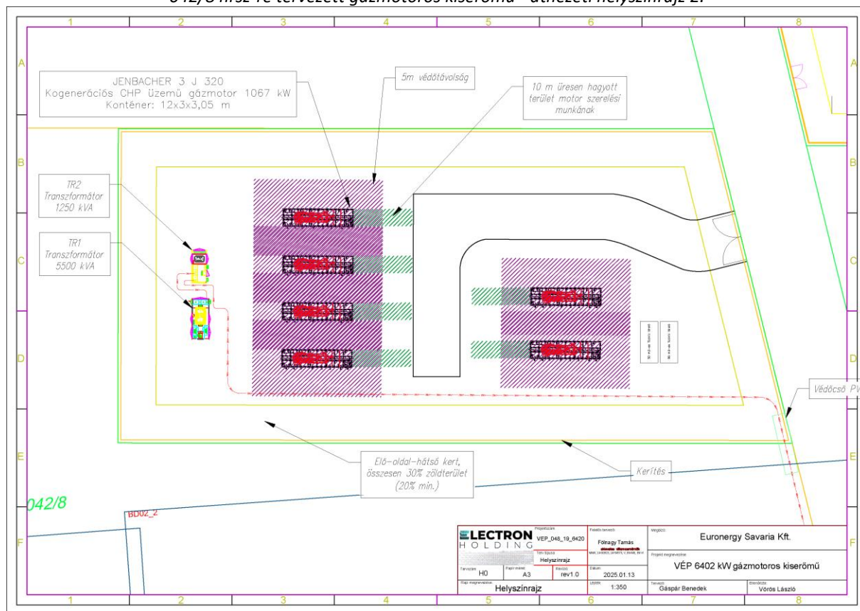
042/8 hrsz-re tervezett gázmotoros kiserőmű - átnézeti helyszínrajz 2.
