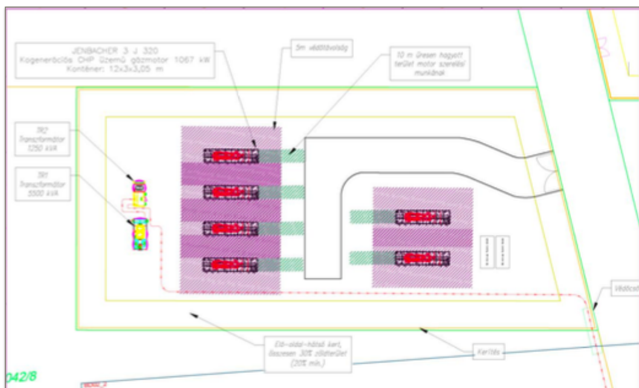
2.4 ábra: A Vép 042/8 hrsz-ú ingatlanon tervezett 6,420 MW teljesítményű gázmotoros kiserőmű felépítése ábrázolva a változással érintett területen
