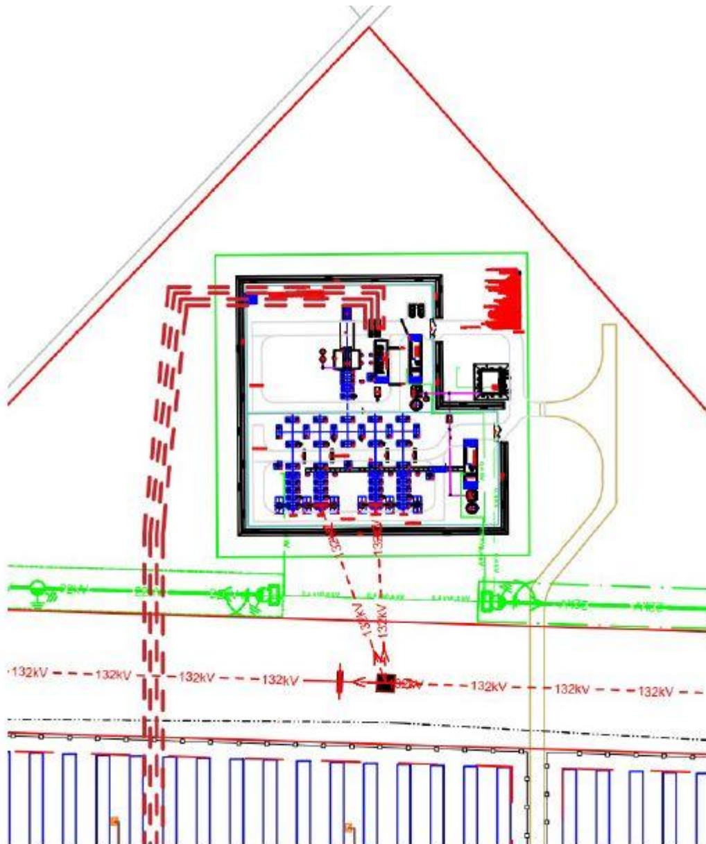
A trafóállomás a meglévő és tervezett 132 kV-os légvezetékek valamint a 132 kV-os tervezett oszlop elhelyezkedése
