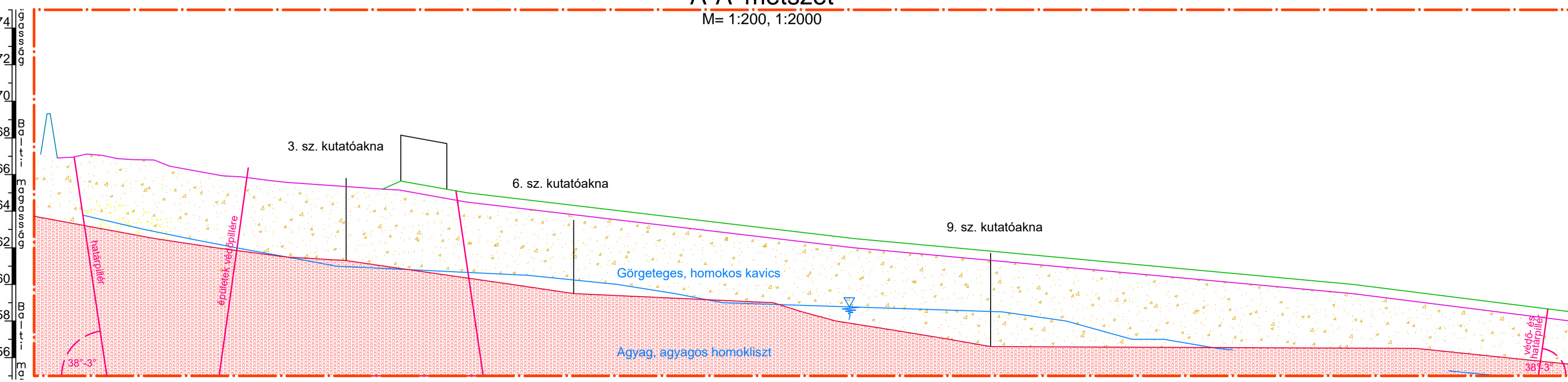
A-A' metszet M= 1:200, 1:2000
