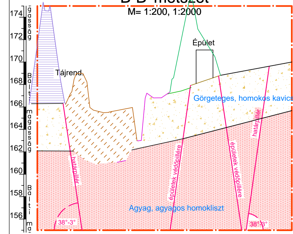
B-B' metszet M= 1:200, 1:2000
