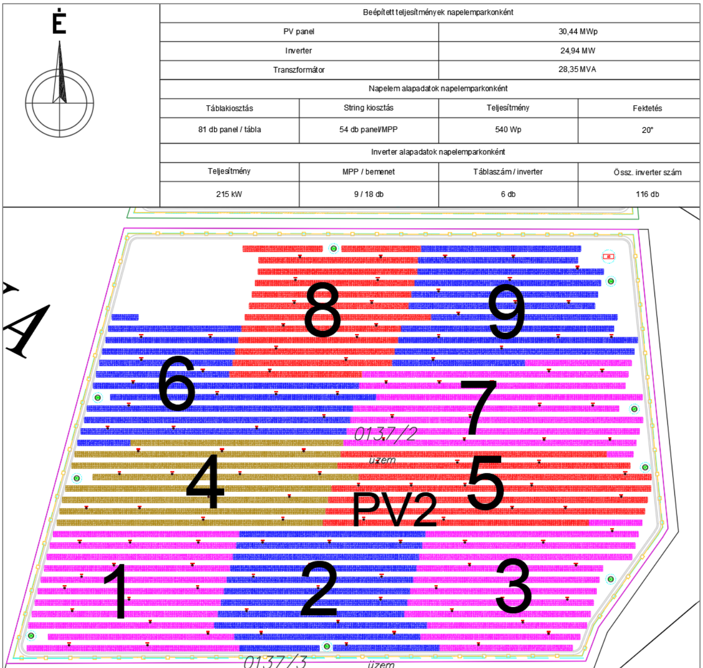
4-1. ábra A naperőmű telepítési elrendezése 20°-os kiosztás esetén
