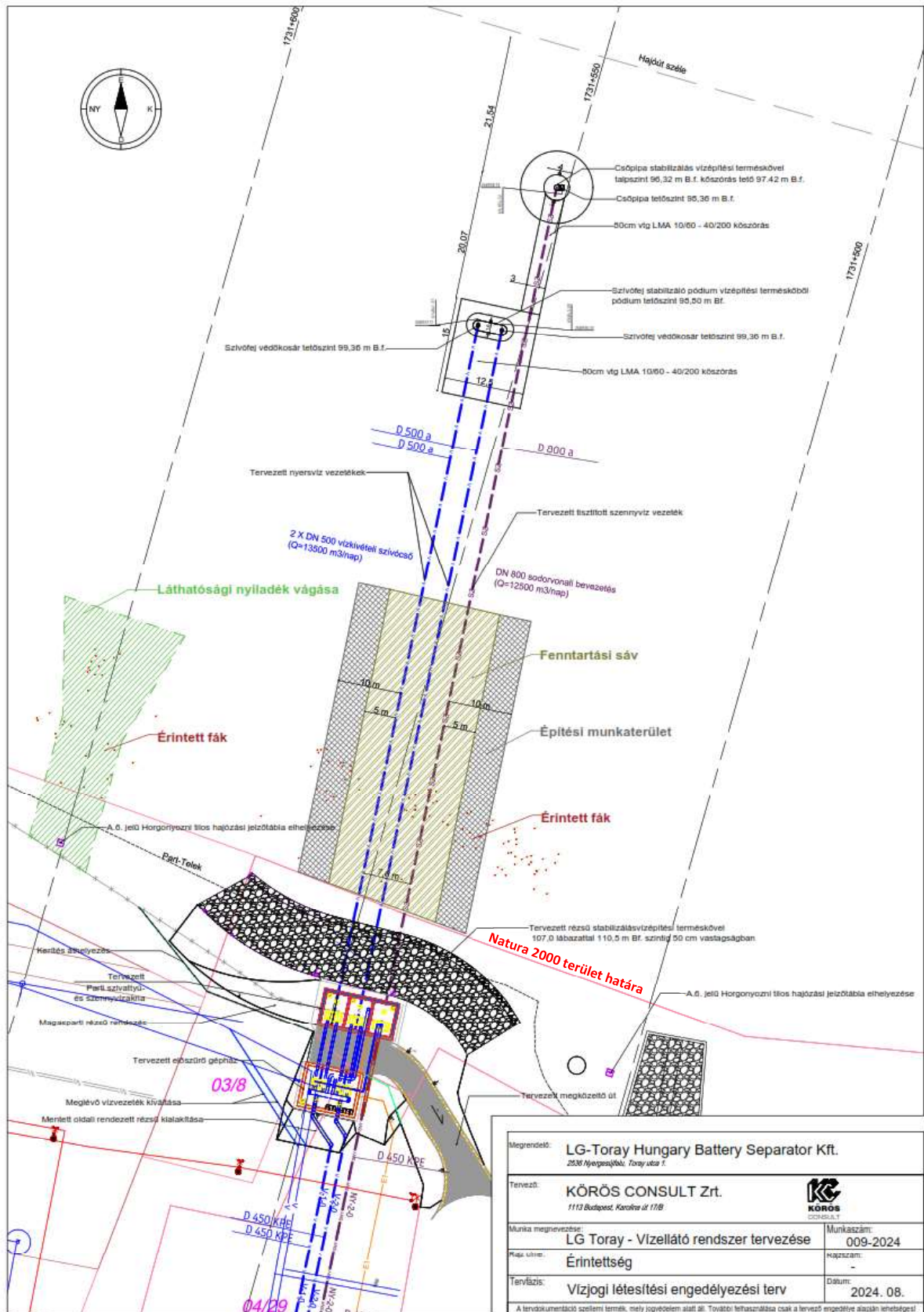
3.3.-1. ábra: Átnézetes helyszínrajz a beruházás Natura 2000 területet érintő részéről
